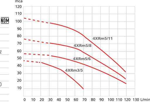
CURVA DE RENDIMIENTO
